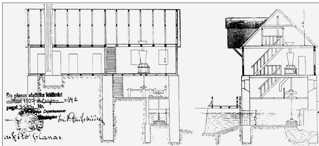
3 pav. Žerkščių–Purvių vandens malūno išilginis ir skersinis pjūviai. Iš LVCA fondų
