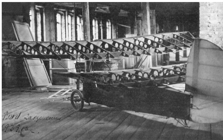
Kapėnų popieriaus fabrike (Mažeikių r.) Vaclovo Tomkevičiaus konstruojamas miniatiūrinis medinės konstrukcijos sportinis lėktuvas „Dangaus blusa“
